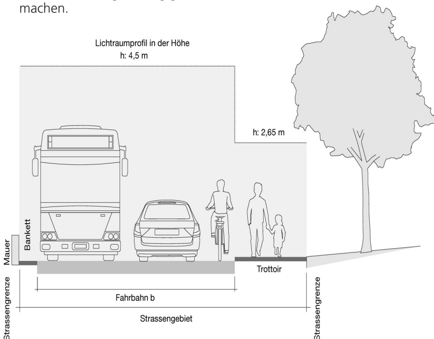
Abbildung: Frei zu haltender Lichtraum gemäss Anhang 5 der Verordnung in Ergänzung zu den Abständen (§ 27 b)
